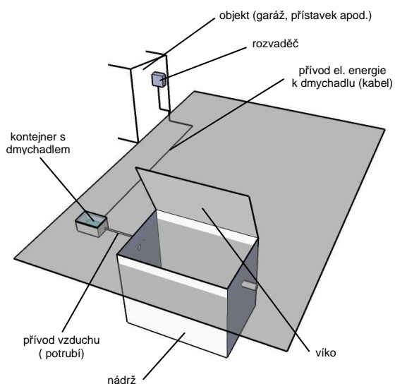
ČOV s rozvaděčem v objektu
